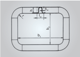
Fig. 7.10 Type XOZ
