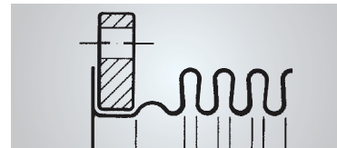
Fig. 3.4 Loose flange
